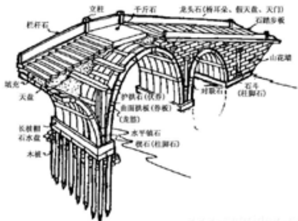
大拱模拟结构示意图
