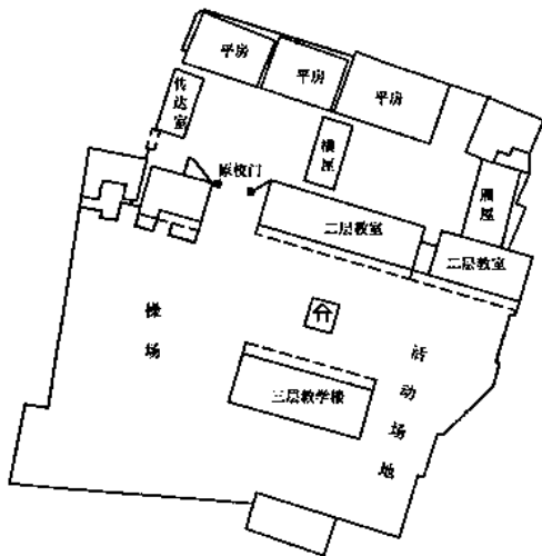
附图五：《丽则女学平面图》
