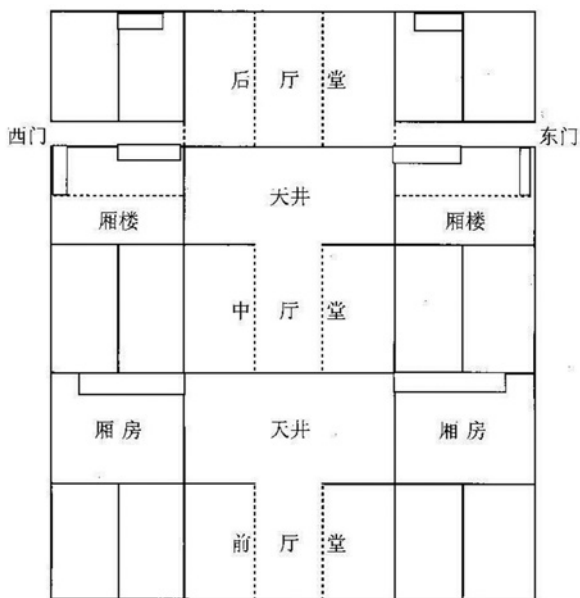
徐氏住宅平面图
